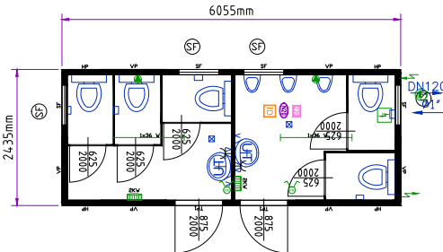
Контейнер-туалет М/Ж 20'
