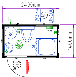
8' контейнер туалет-душ
